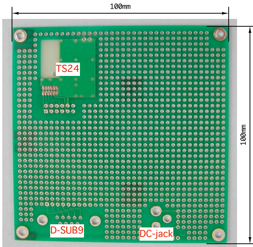
部品面
