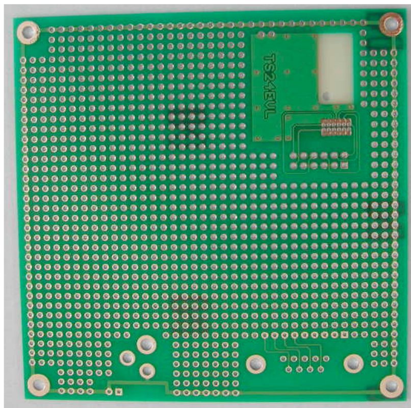
半田面
